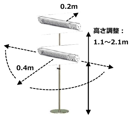
図：スタンド設置の場合の離隔距離
